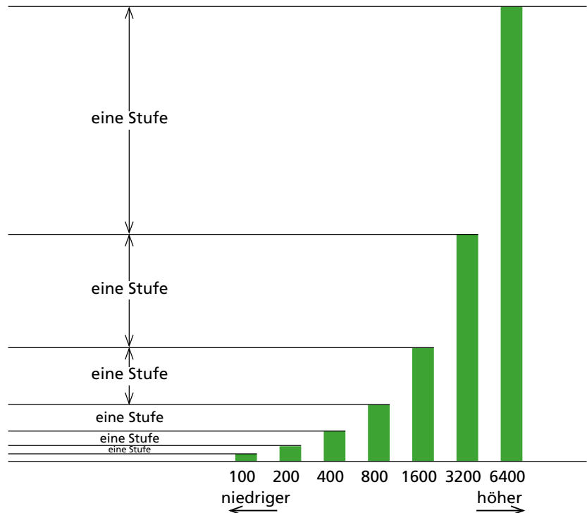
ABBILDUNG 2.10 Der ISO-Wert gibt den Pegel des digitalen Sensorsignals wieder – je höher der Wert, desto größer die Verstärkung. Meist wird die ISO-Empfindlichkeit bei abfallender Beleuchtungsintensität erhöht.
